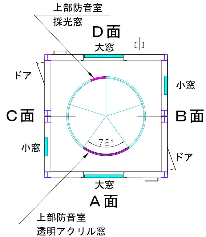
平面図
