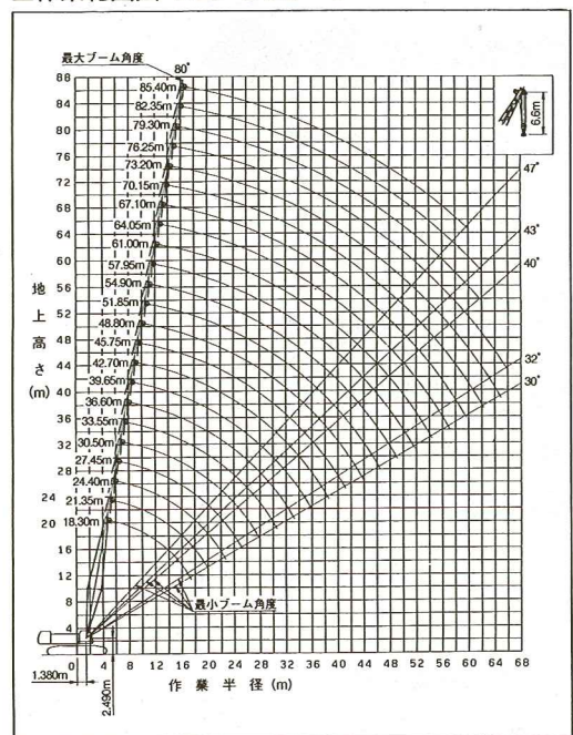
■作業範囲図 クローラークレーン
