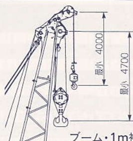
ブーム・1m補助ジブ
