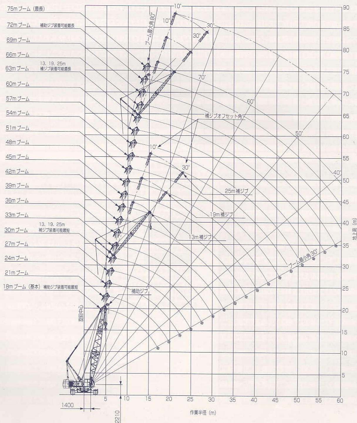
補ジブ
