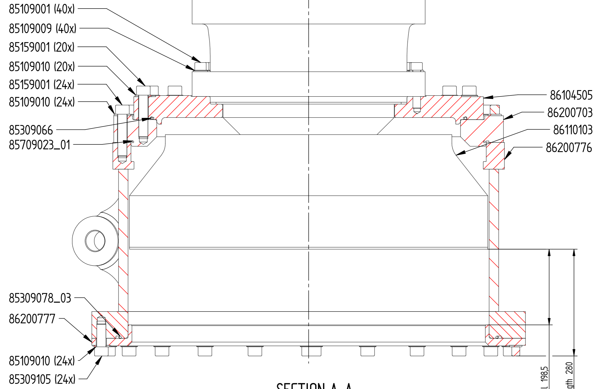
SECTION A-A 1:5
