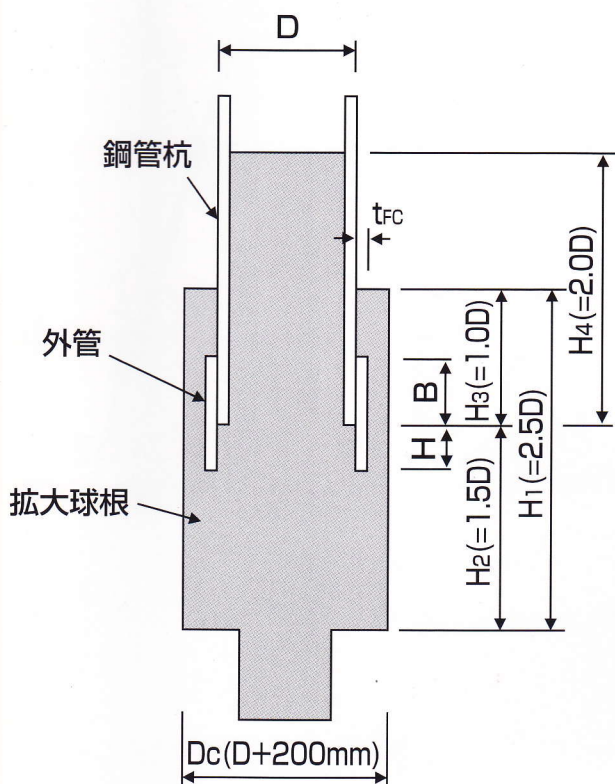
■杭先端部の概念図
